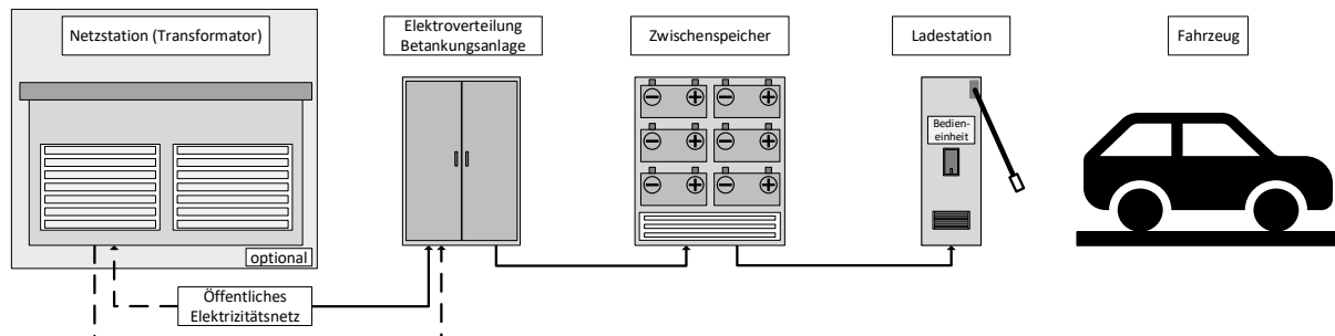
Abbildung A2-3: Einrichtungen der Elektromobilität mit Zwischenspeicher (Gleichstrom-Ladung)
