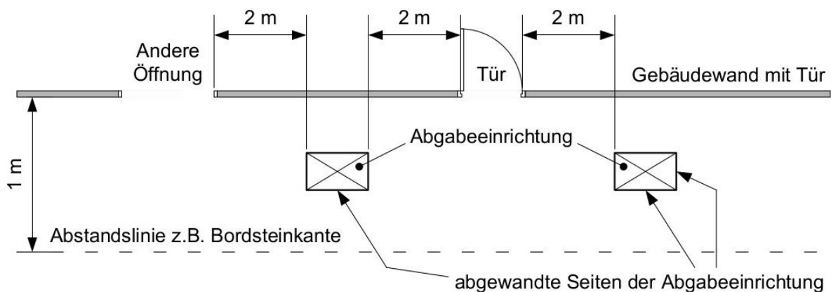
Abbildung 1: Zu Öffnungen in Gebäuden abgewandte Seiten von Abgabereinrichtungen
