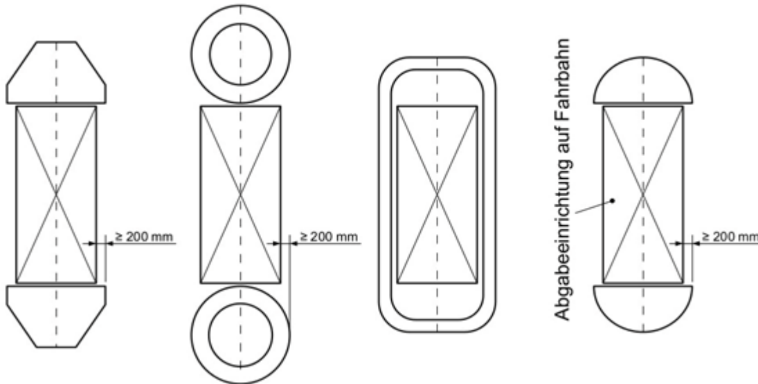
Abbildung 2: Anfahrerschutz an Abgabereinrichtungen
